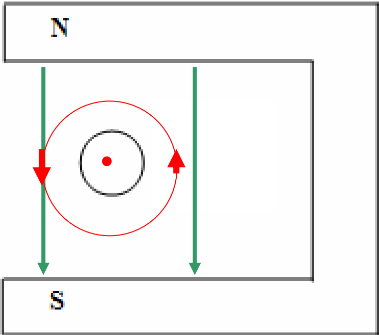
Verlauf der Feldlinien des Leiters
